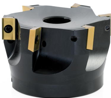
ATTACCO A MANICOTTO - Shell Shank
