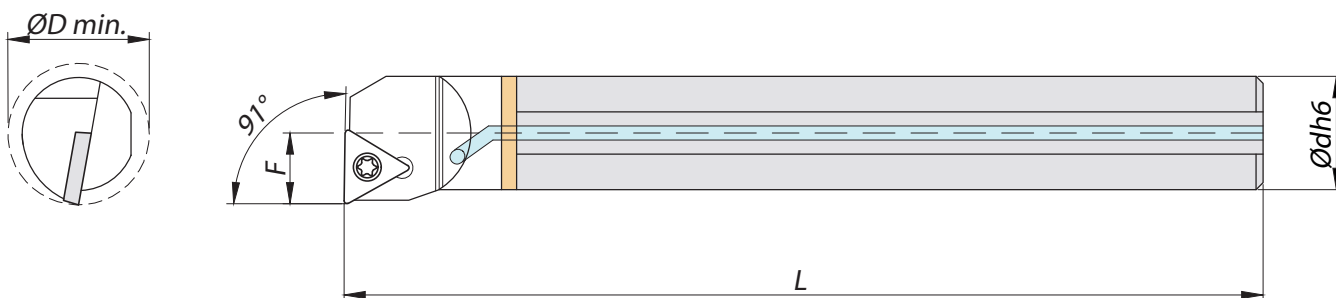
ATTACCO CILINDRICO CON PIATTO PARALLELO - Cylindrical Shank with Flat
