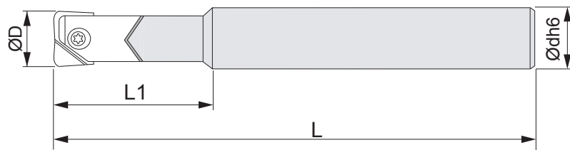
ATTACCO CILINDRICO IN METALLO DURO - Carbide Cylindrical Shank
